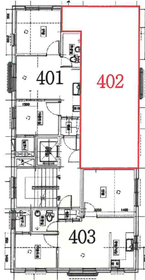
(호별배치도)
