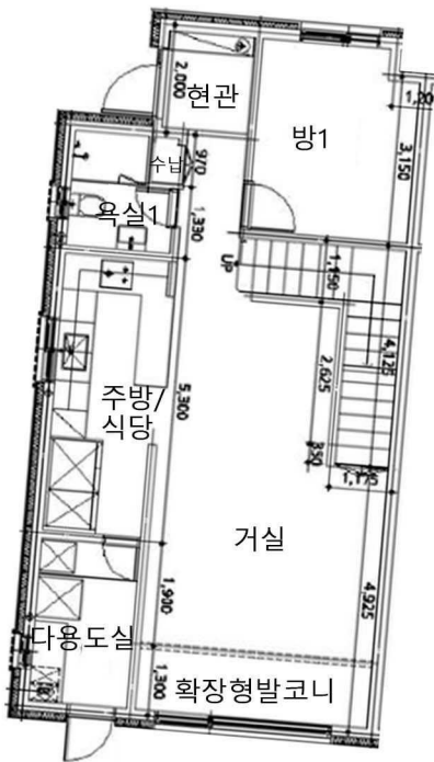
< 102호 : 하부층(1층) >
