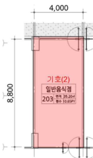
< 내부구조도 >
