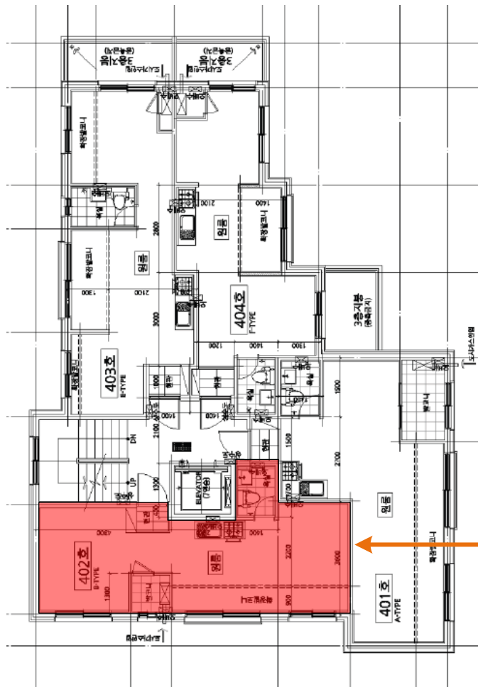
[호별배치도]
