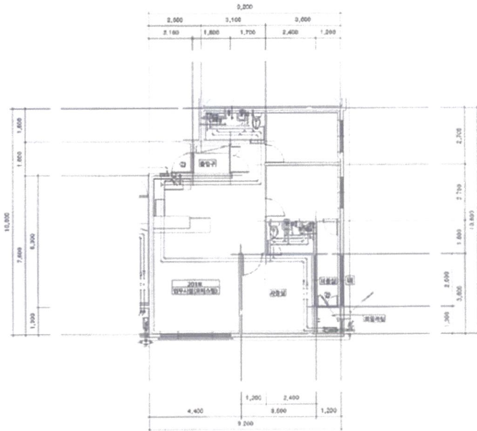
<내부구조도>
