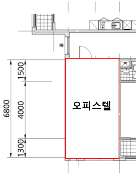
[내부구조도] 제5층 제515호
