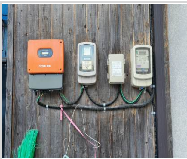
태양광발전설비
