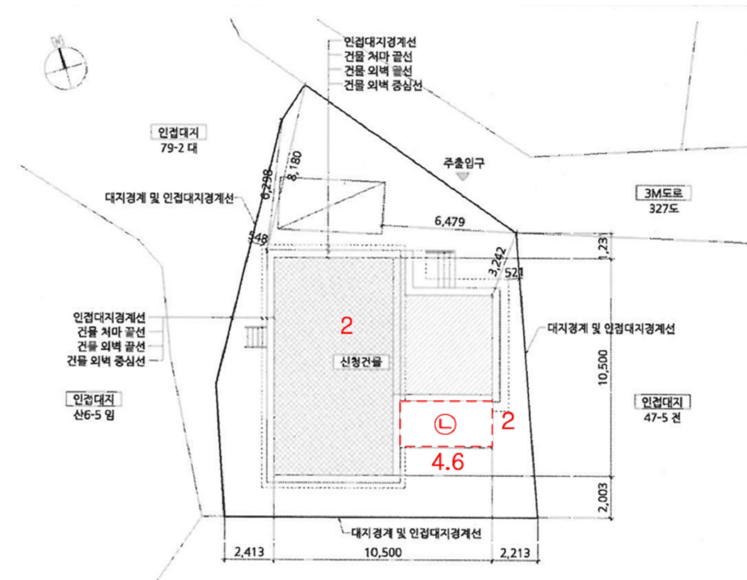
2. 배치도
