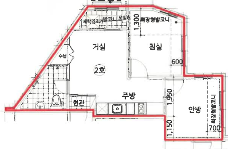
<내부구조도>
