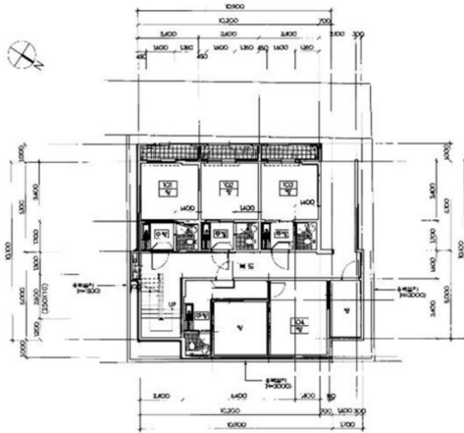
[기호(2) 건물 지하1층]
