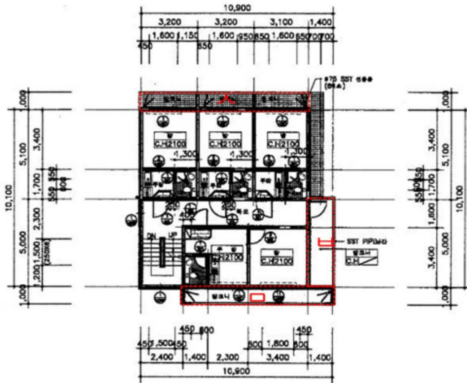
[기호(2) 건물 3층]
