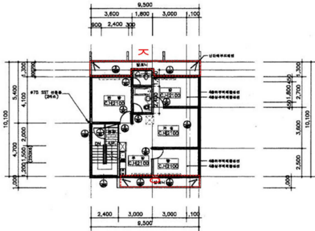
[기호(2) 건물 4층]
