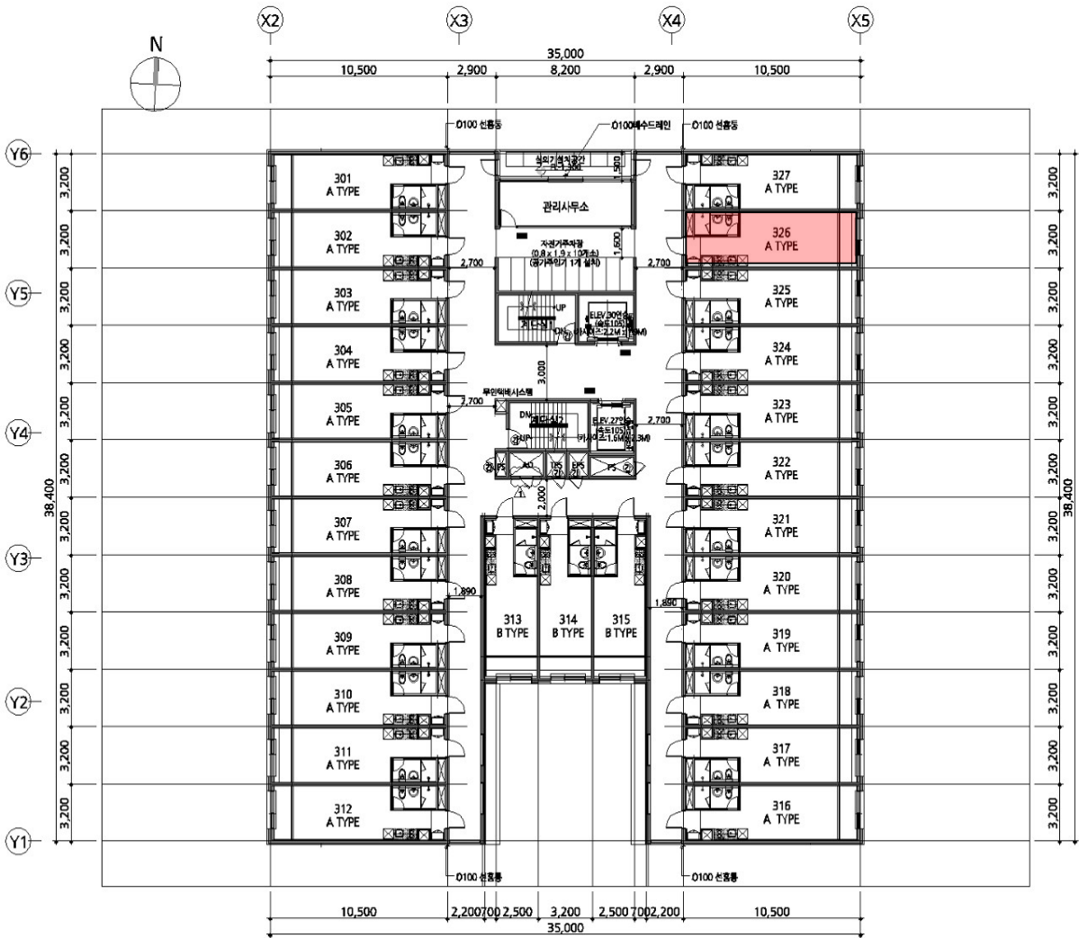
1 3층 평면도 축척: 1/200(A3)
