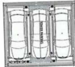
< 본건 제5층 호별배치도 >
