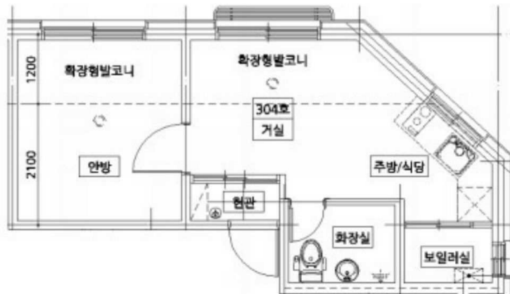
제3층 제304호 (건축물 현황도)
