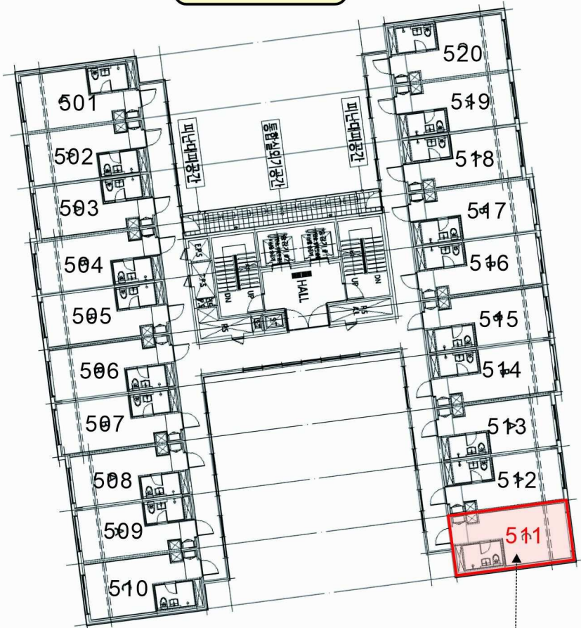
호별 배치도
