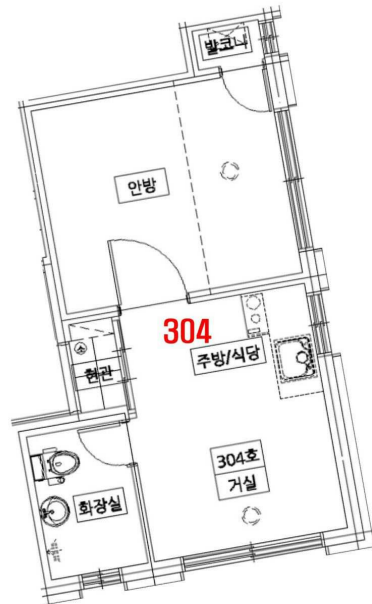
< 내부구조도 >
