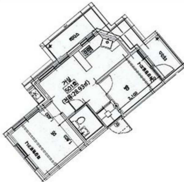
< 본건 제5층 제501호 내부구조도 >
