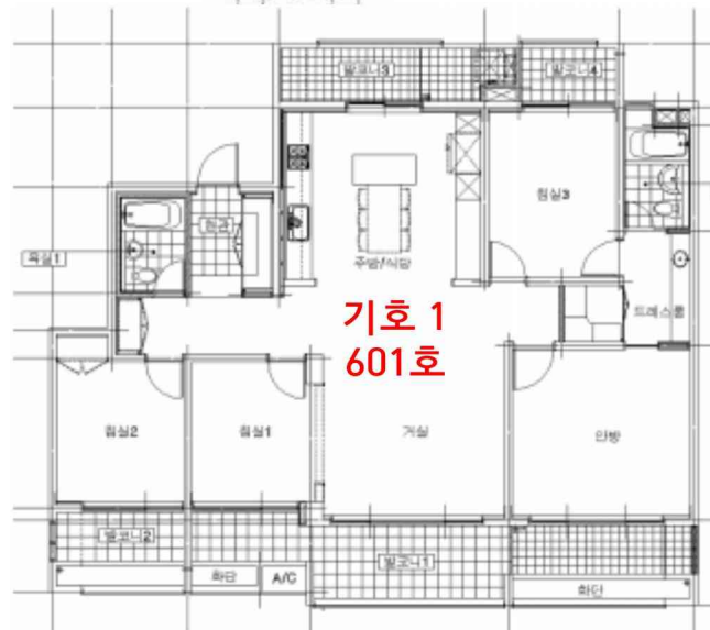
【6층 호별배치도 및 내부구조도】
