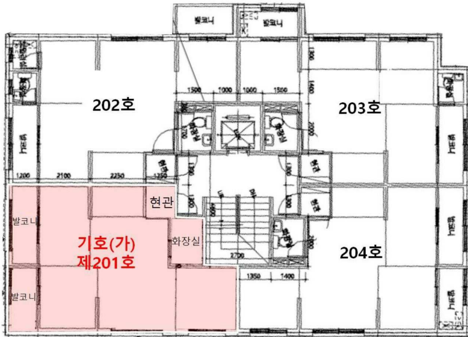
< 제102동 제2층 호별배치도 >
