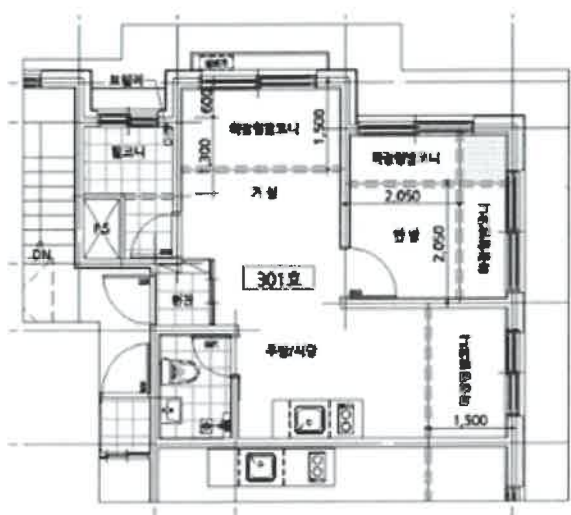
< 내부구조도 >
