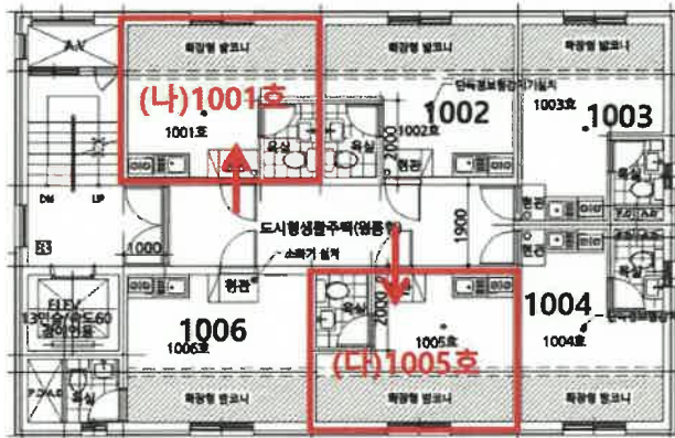
[10층 평면도]
