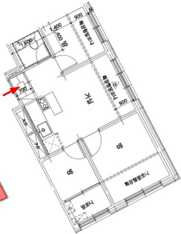
[내부구조도]
