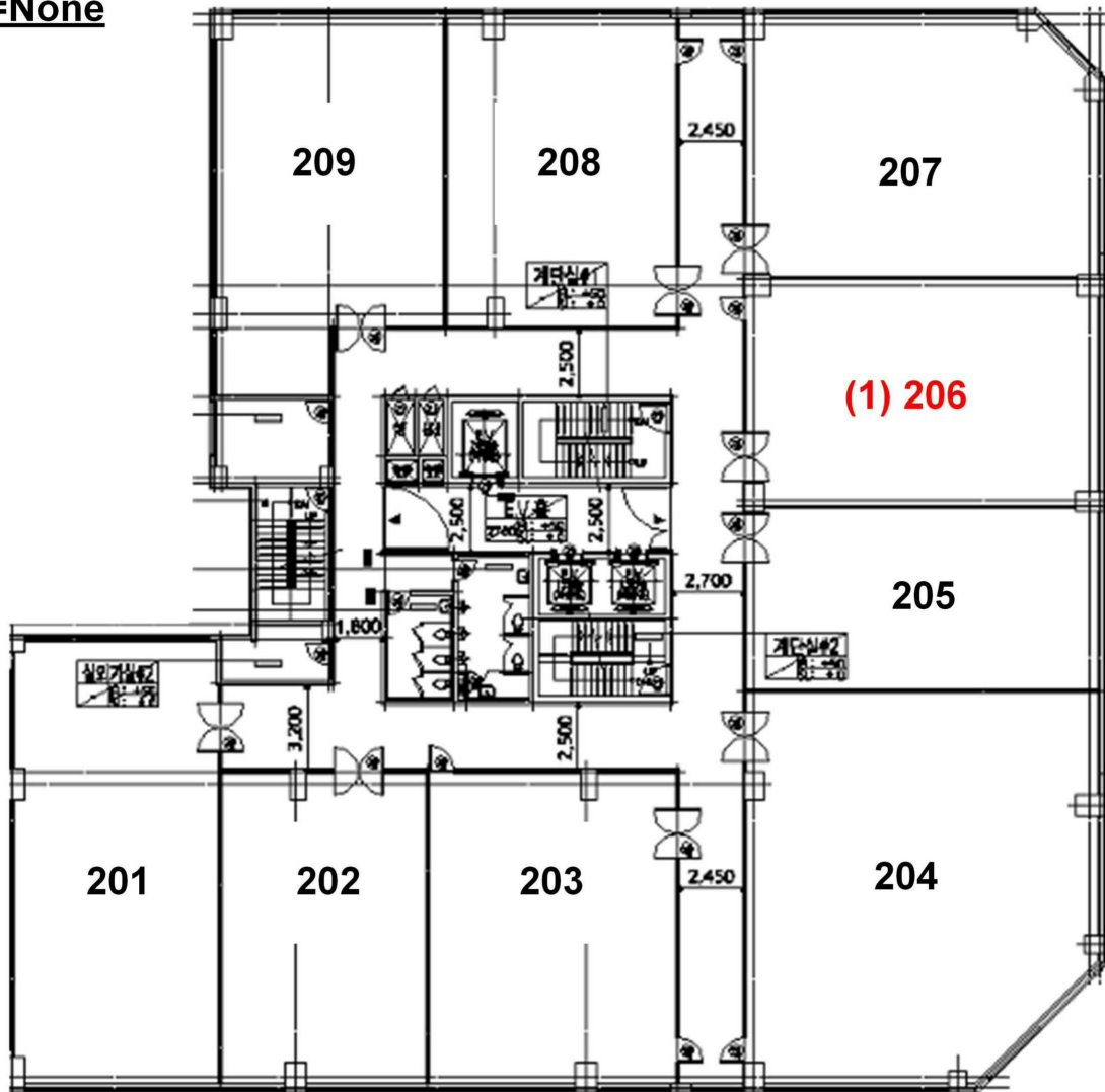
명지동 3593-1, 우진메디컬프라자 2층 호별배치도
