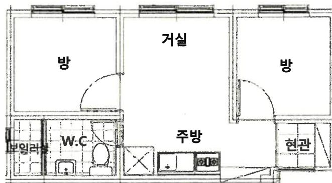
< 내 부 구 조 도 >
