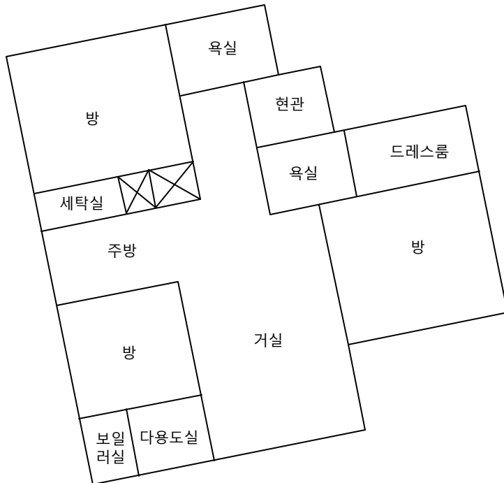
제1502호 내부구조도
