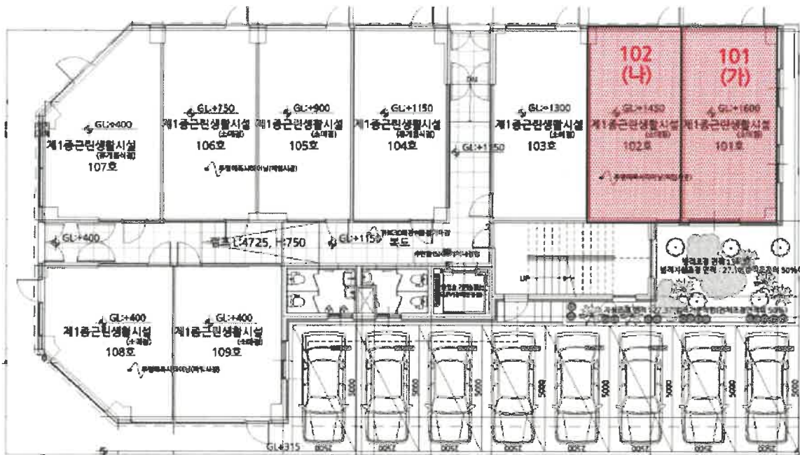
[ 비발디시티 1층 호별배치도 ]
