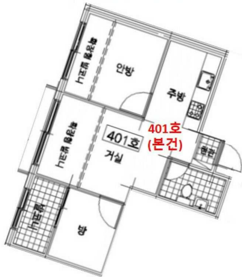
내부구조도
