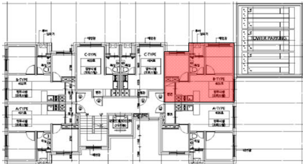
층별현황도 (4층)
