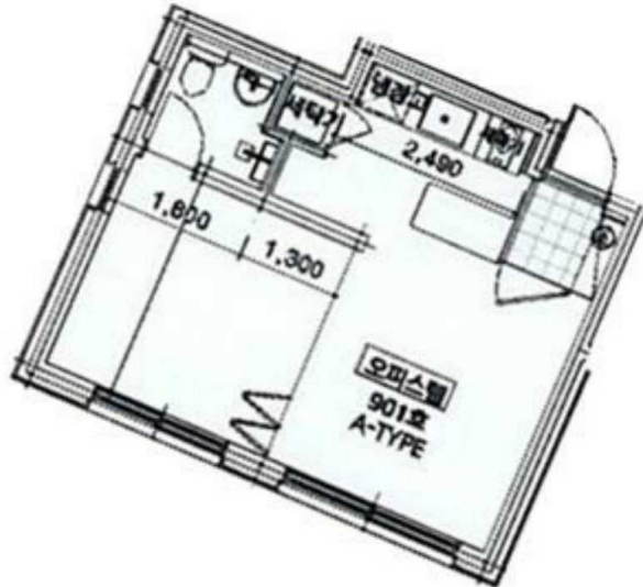
< 본건 제9층 제901호 내부구조도 >
