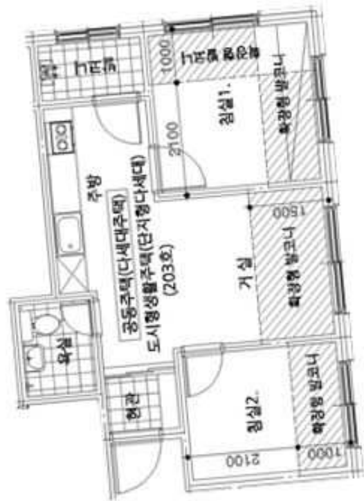
<내부구조도>
