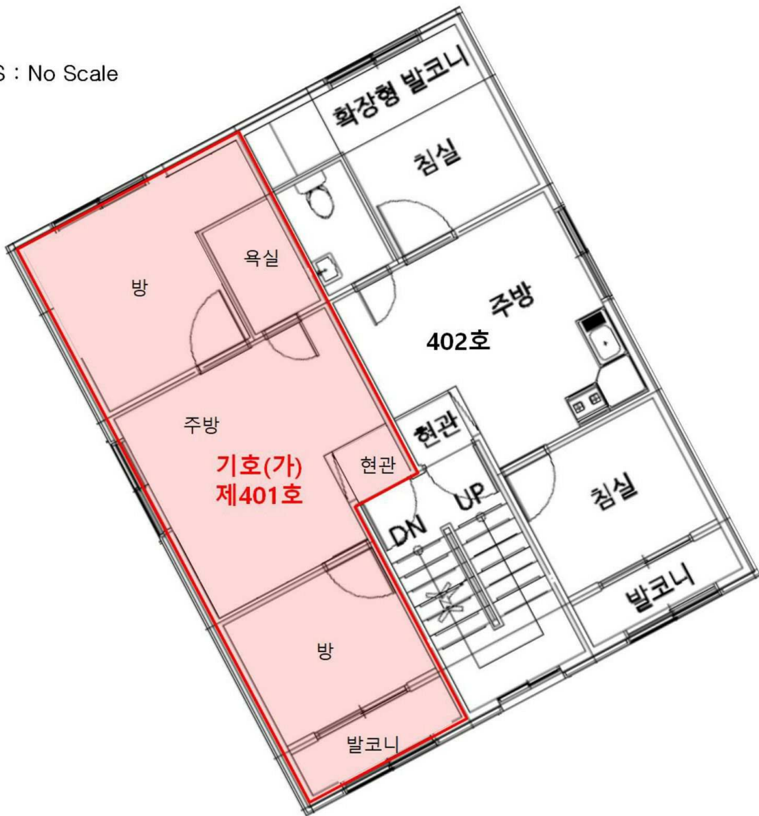
< 제4층 호별배치도 및 내부구조도 >
