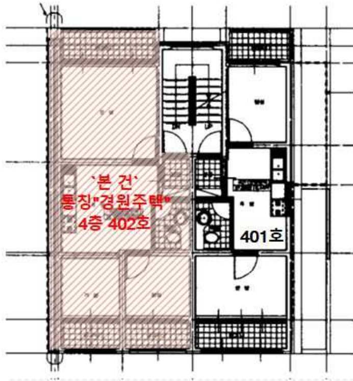
4층 호별배치도
