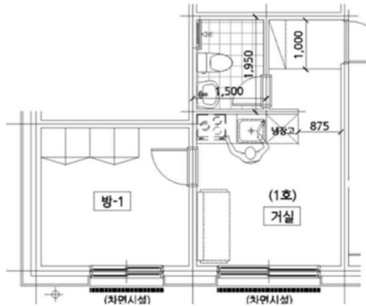
내부구조도
