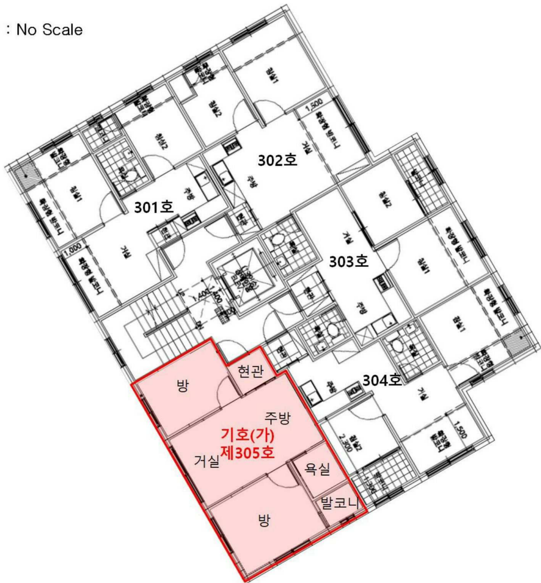
< 제3층 호별배치도 및 내부구조도 >
