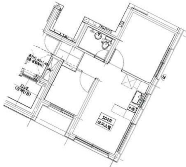
504호 평면도
