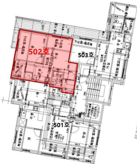
<제5층 호별배치도>
