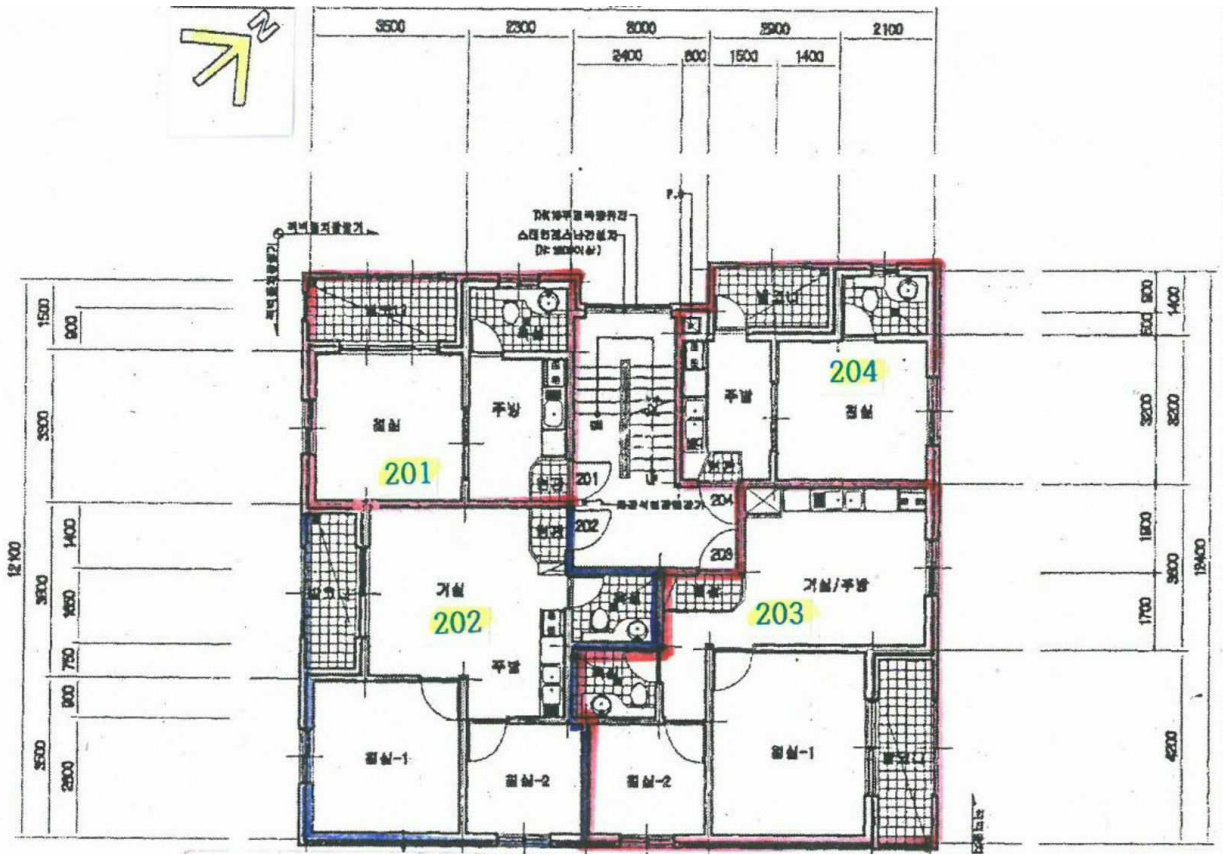
2층 평면도
