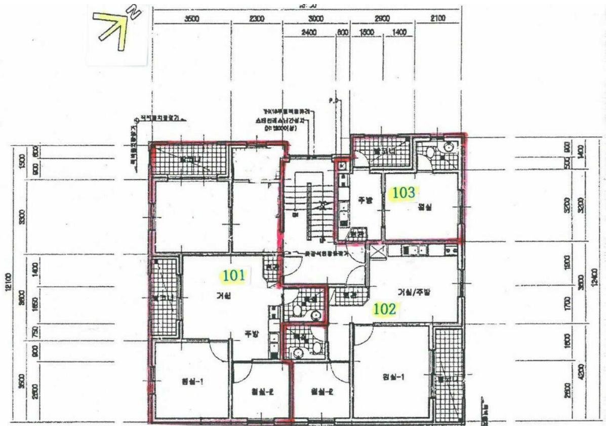
1층 평면도
