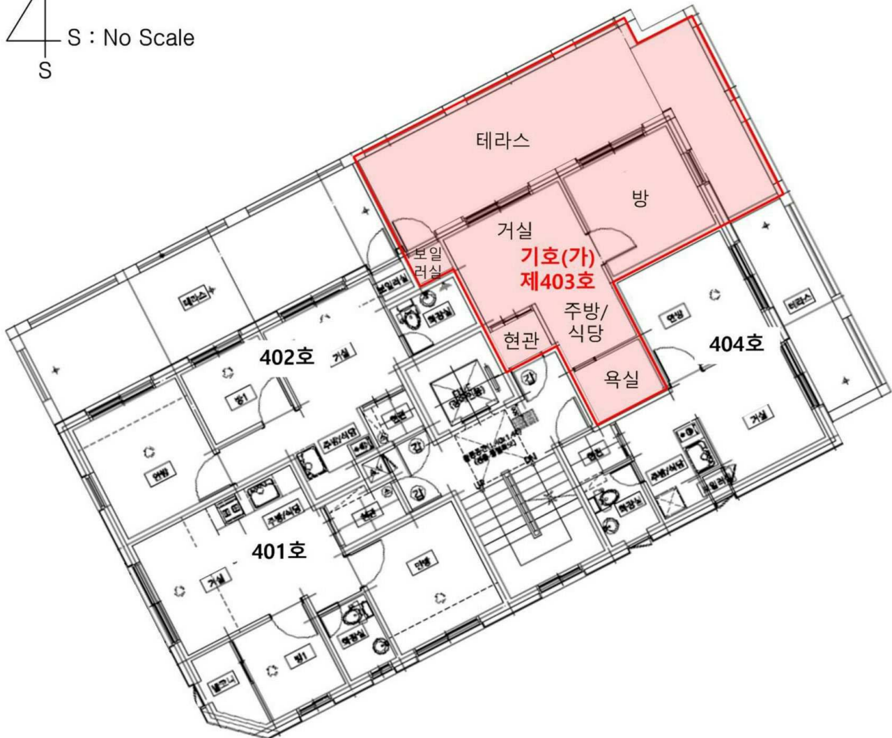
< 제4층 호별배치도 및 내부구조도 >
