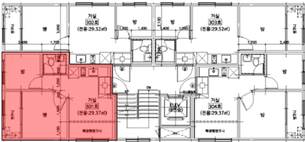
층별현황도 (3층)
