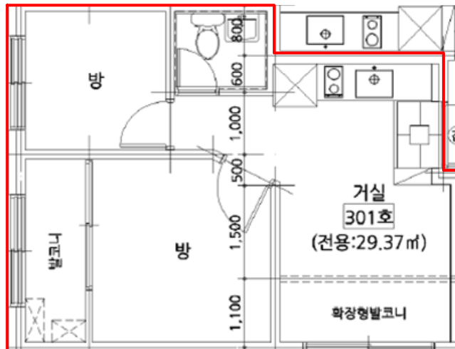
내부구조도 (301호)
