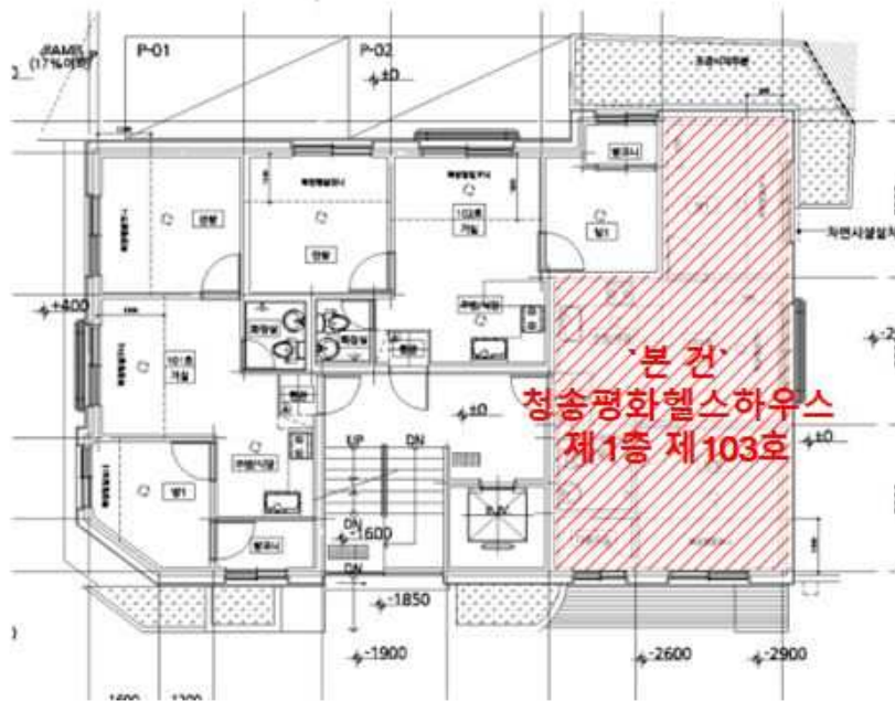
내부구조도(1층 103호)
