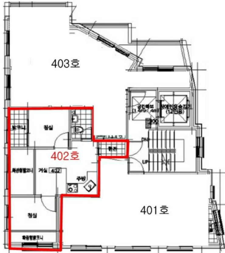
< 삼원아이빌비 4층 배치도 및 402호 내부구조도 >
