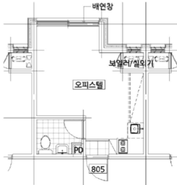
호별배치도
