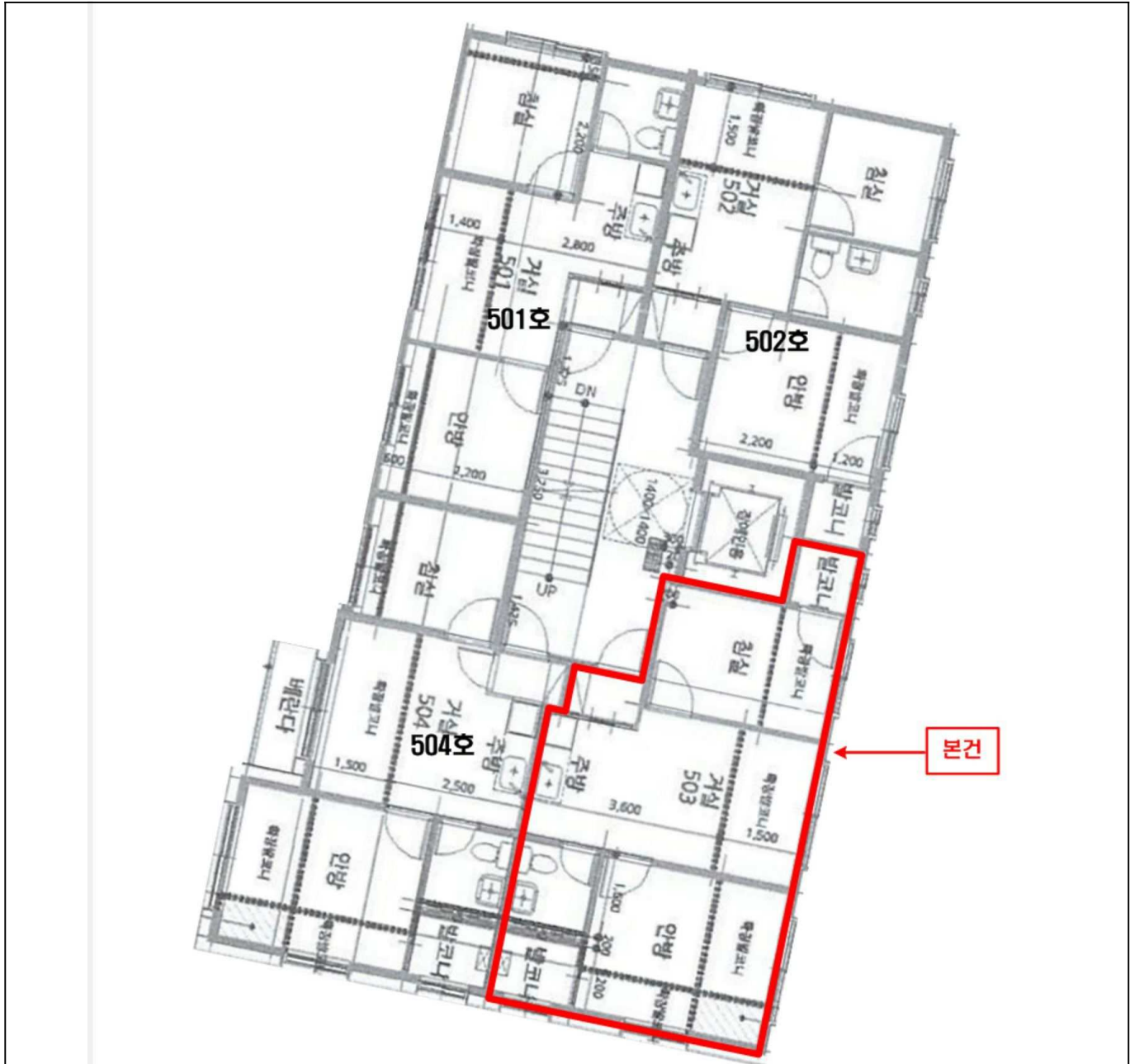
< 호별배치도 및 내부구조도 >
