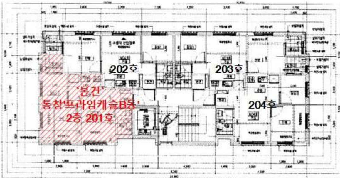
지상 2~5층 평면도 44-V-102
