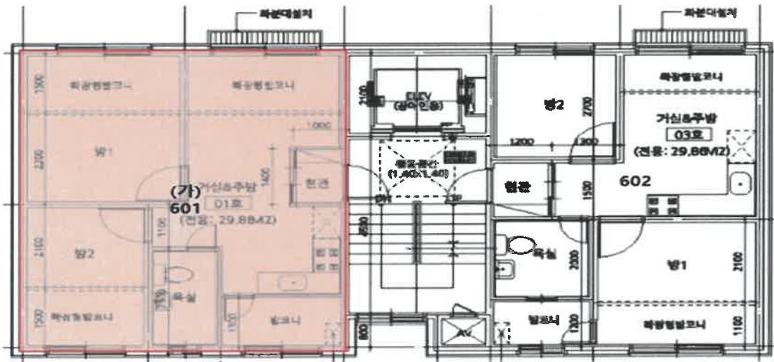
< 호별 배치도 >
