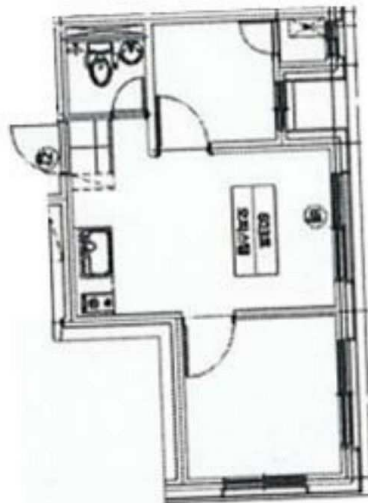
< 본건 제6층 제603호 내부구조도 >
