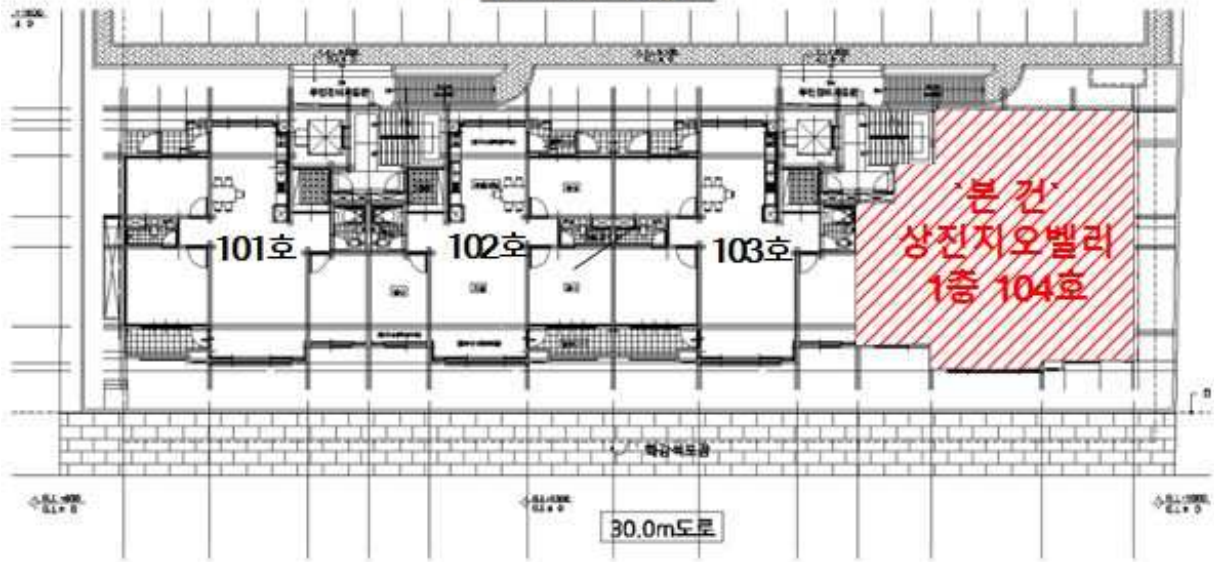
1층 호별배치도
