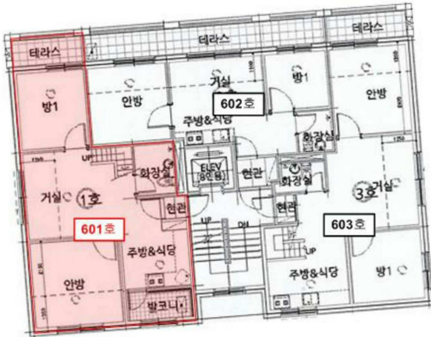
< 본건 남성아트빌 제6층 호별배치도 >
