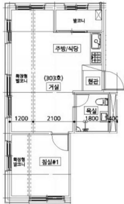
제3층 제303호 (건축물 현황도)
