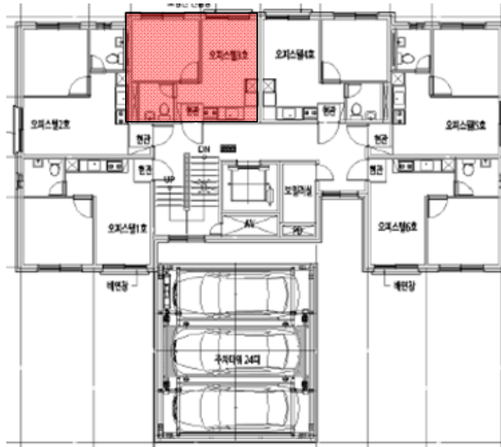
층별현황도 (4층)
