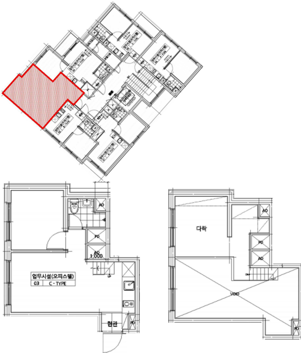
제6층 제603호 (건축물현황도)
